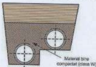
Instalare țevi paralele în tranșee în trepte
