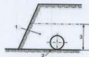
Fig. A6.9 Condiția de pozare 3
